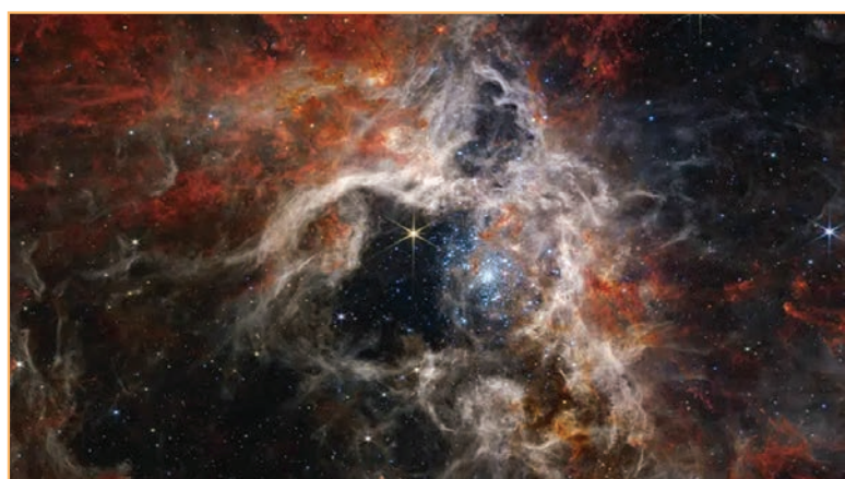
蜘蛛星雲 (Tarantula Nebula) : 距離地球 161,000 光年，那裏誕生了成千上萬個恆星
